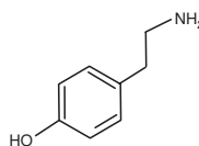
Tyramine
